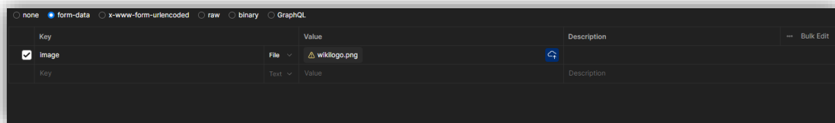
ábra 72: kérés törzse
