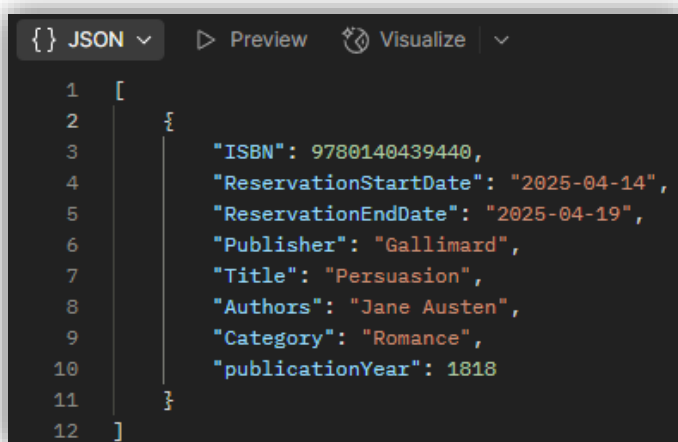
ábra 94: válaszüzenet
