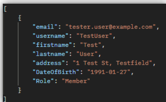
ábra 31: válaszüzenet
